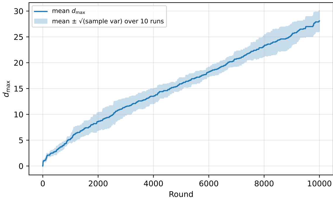
d_{\max} vs round (MovieLens)
