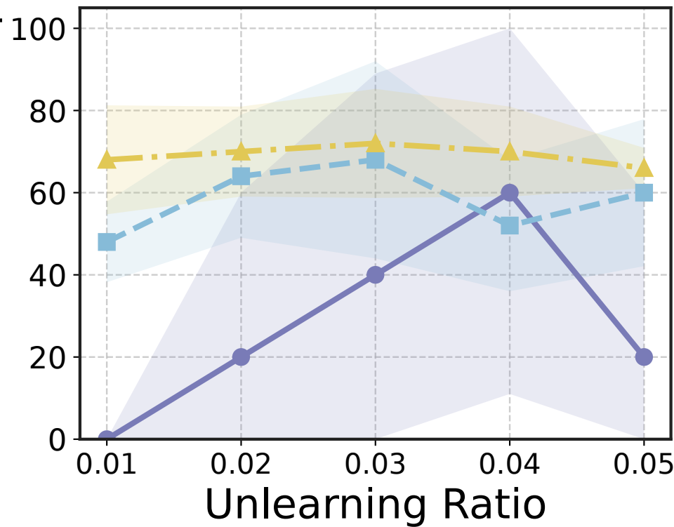
FedU
