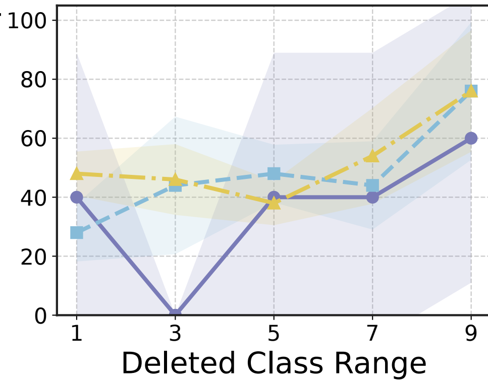
FedU
