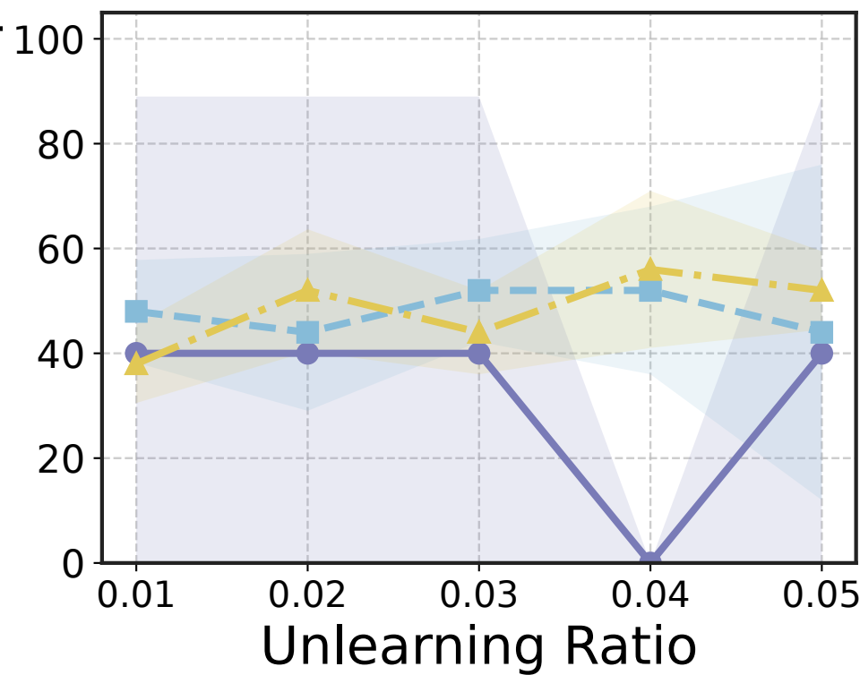
FedU
