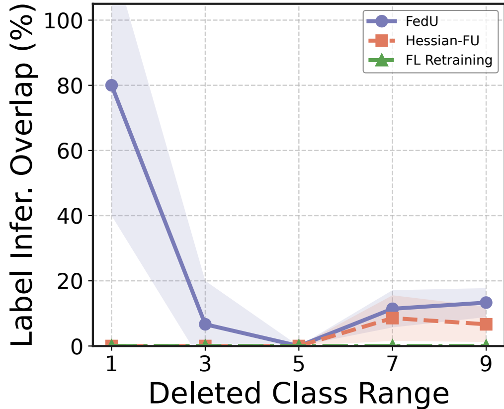
CrossLeak
