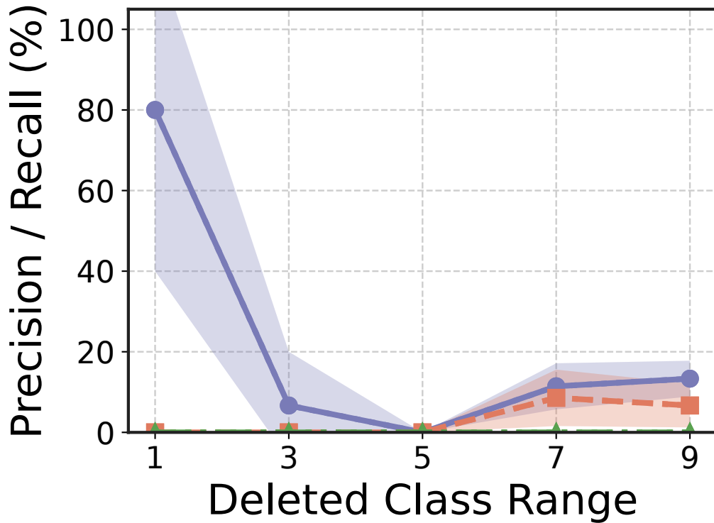
CrossLeak
