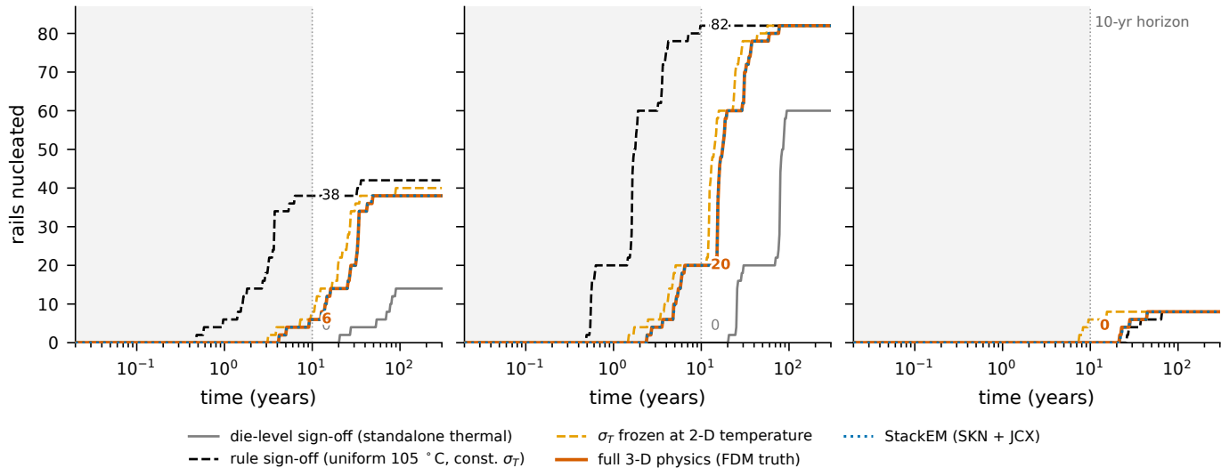
D1 (IO, 2 W)
