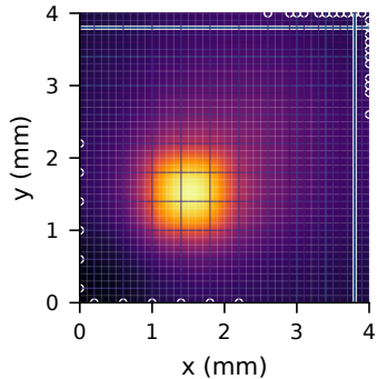
D1 (2 W) earliest 9.87 yr
