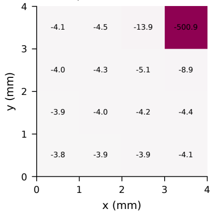
power blocks of D1
