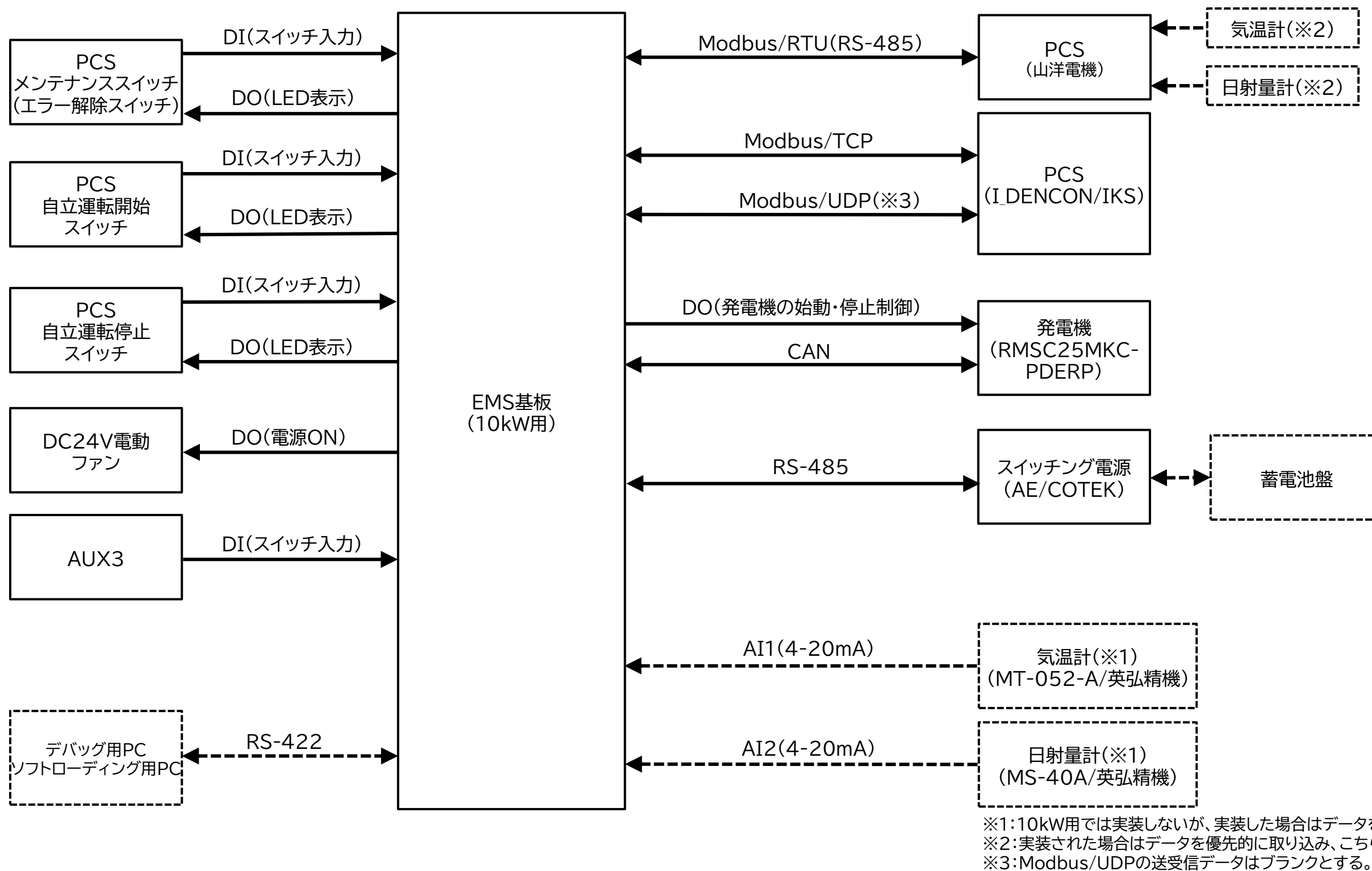
図2.1.1 システム構成図
