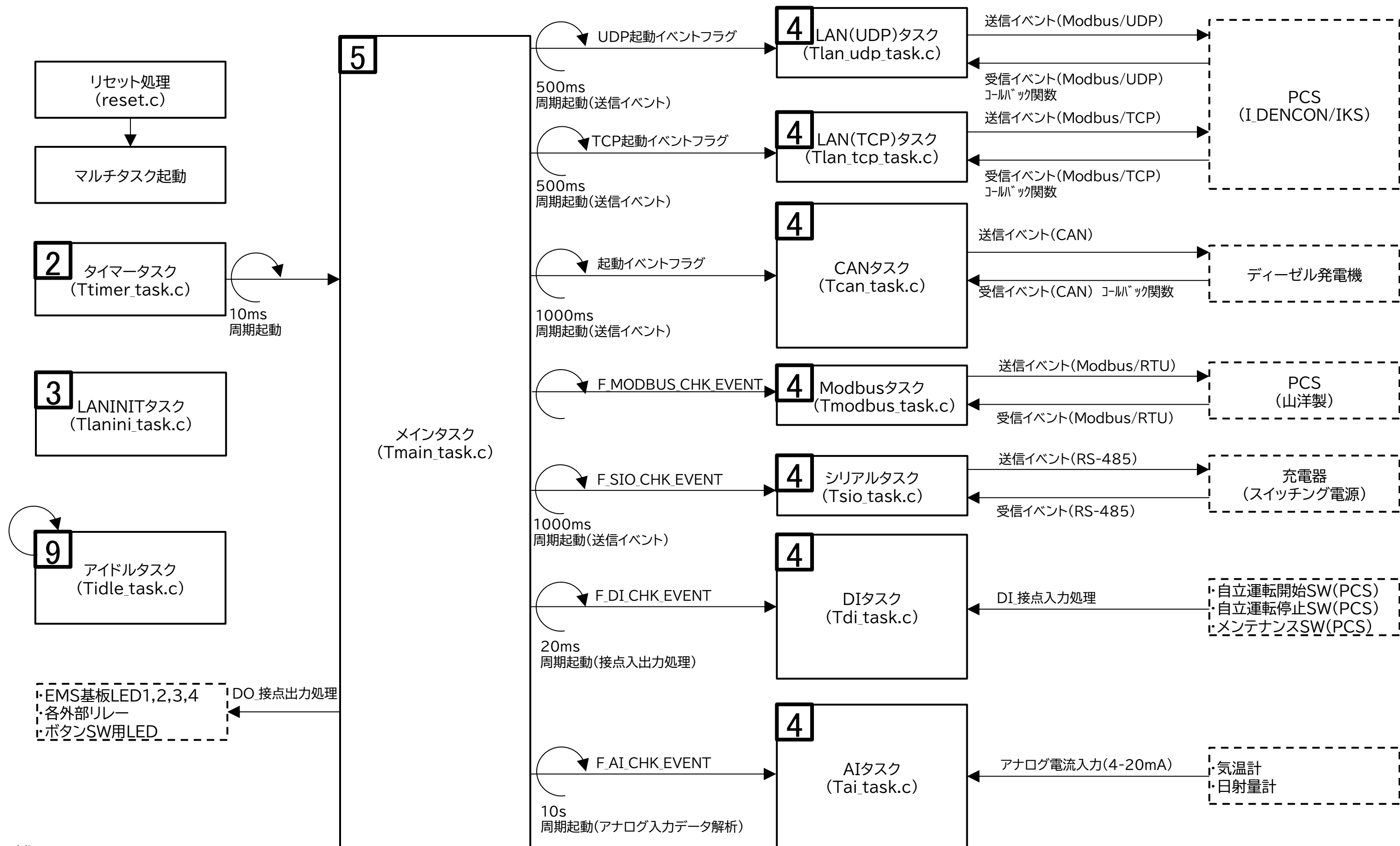
図3.1.1 タスク構成図
