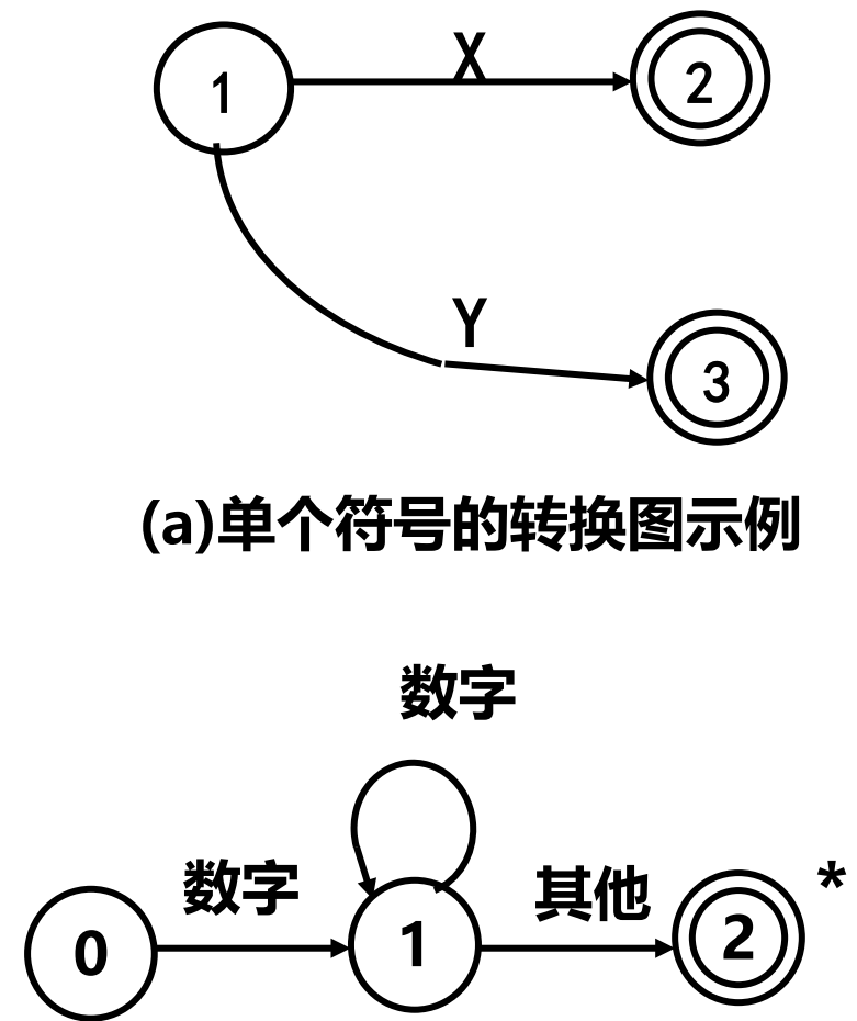
(c) 识别整数的转换图
