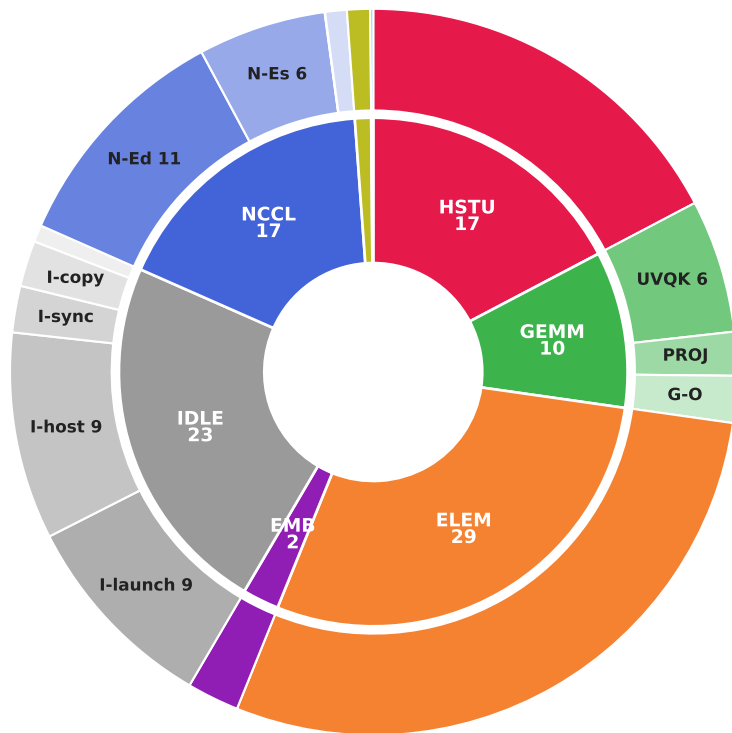
v26.05 (median 94.0 ms/step · MFU ~16%)
