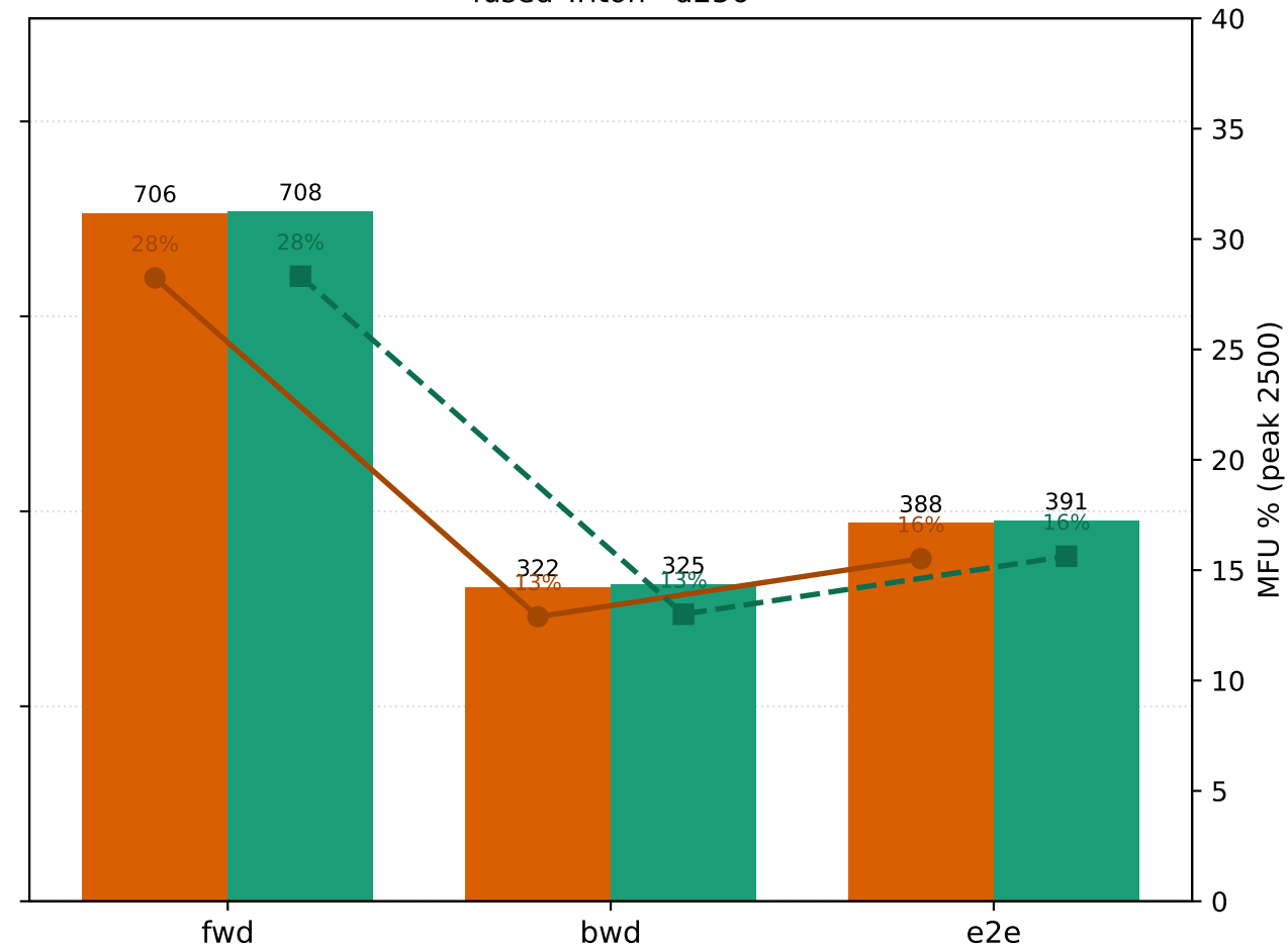
fused Triton · d256
