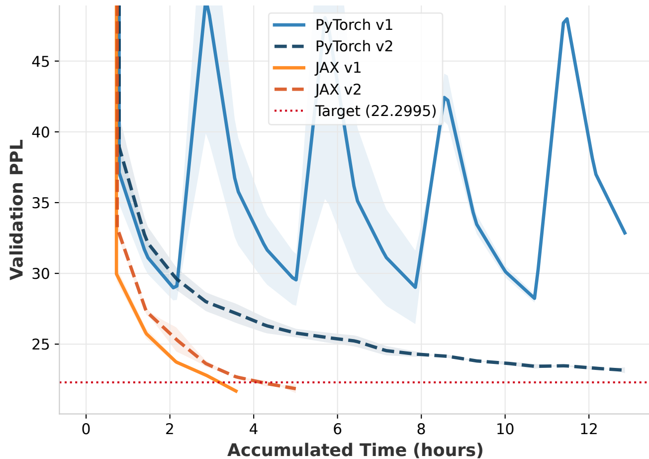
Workload: finewebedu_lm (Metric: ppl)
