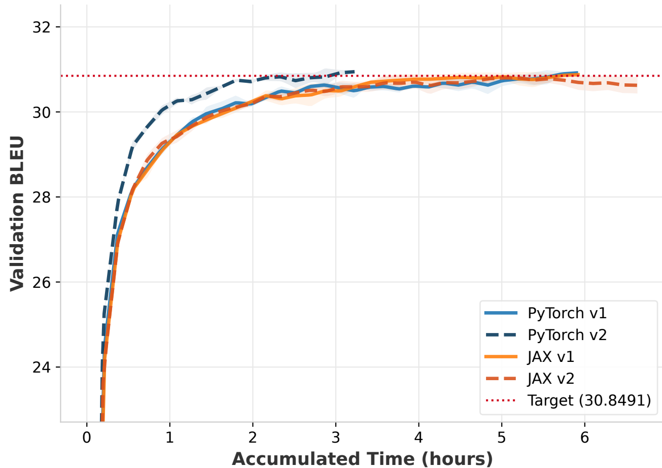
Workload: wmt (Metric: bleu)
