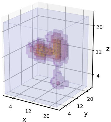
ref9
