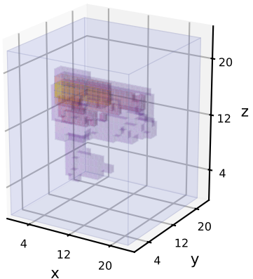
ref3
