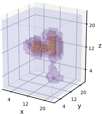
ref9
