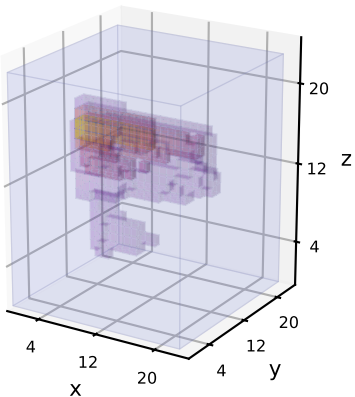
ref3
