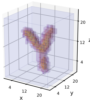
BP
