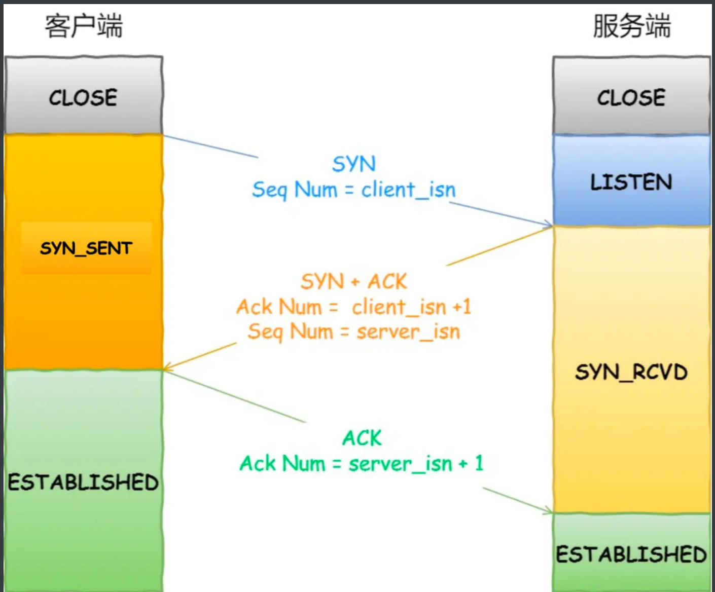
TCP 三次握手
