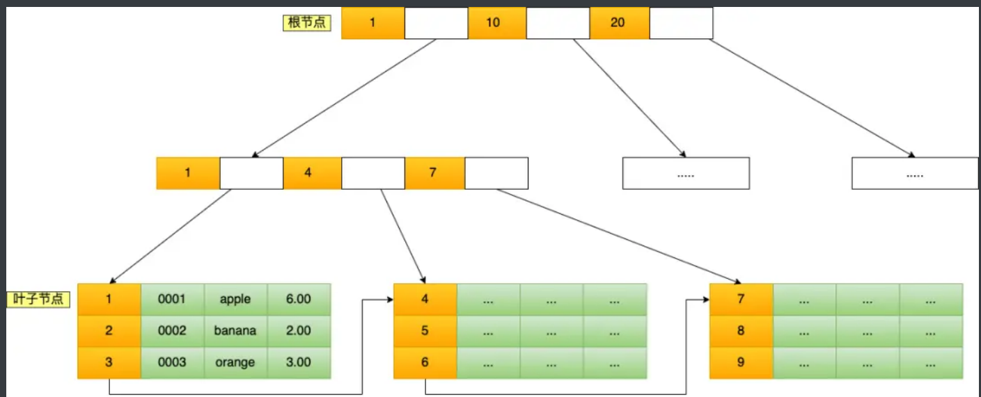
主键索引 B+Tree
