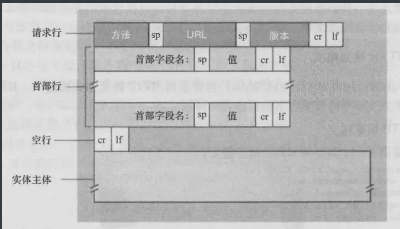
HTTP 请求报文结构
