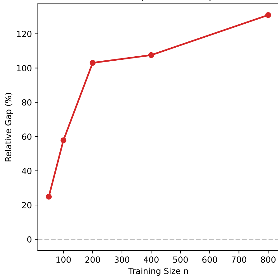
(d) Sample Size \rightarrow Gap
