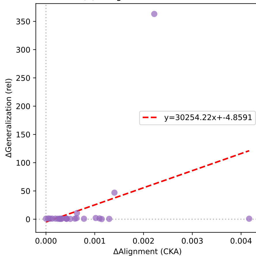
(e) \Delta\text{Align} vs \Delta\text{Gen} r=0.367
