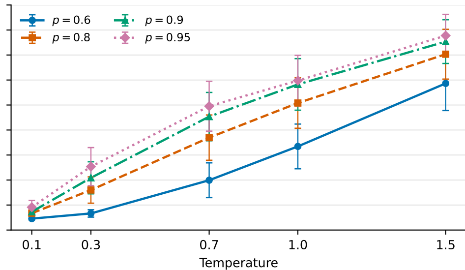
Pure top- p
