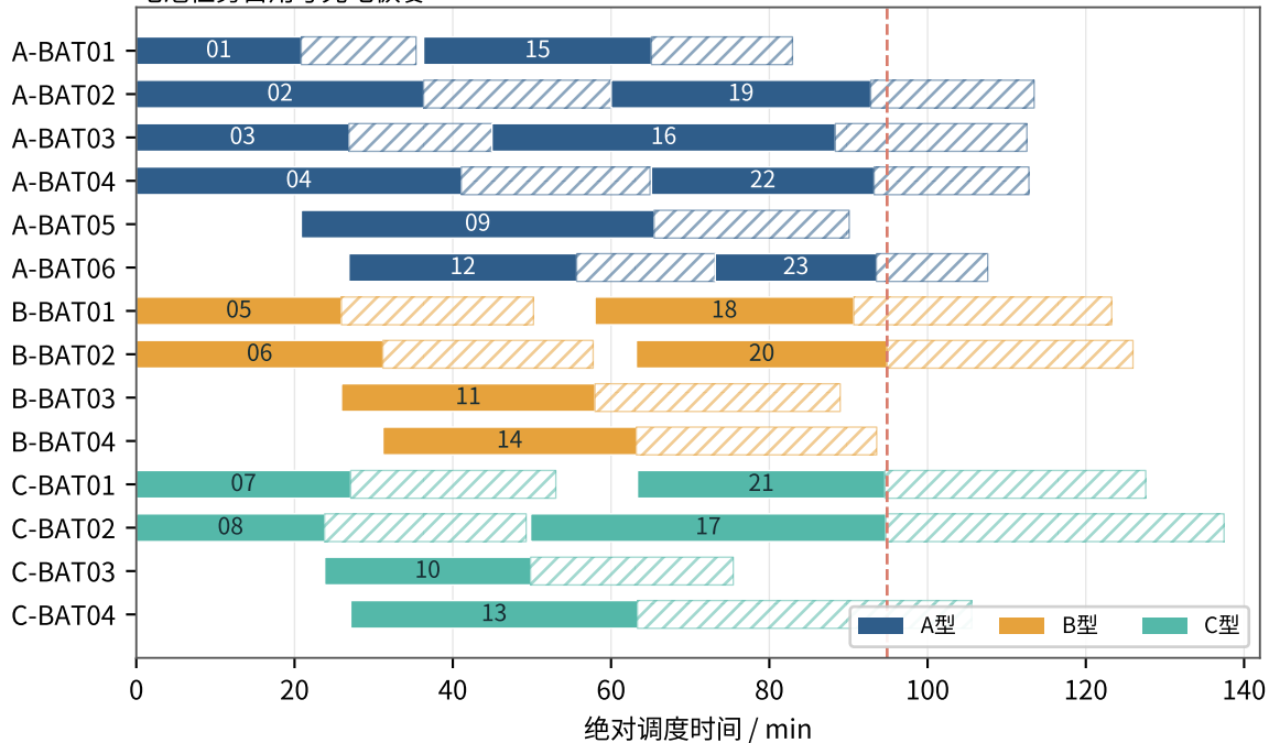
电池任务占用与充电恢复
