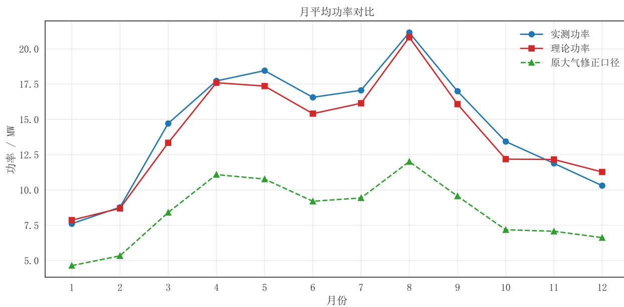
图 2: 月度实际功率与理论功率对比
