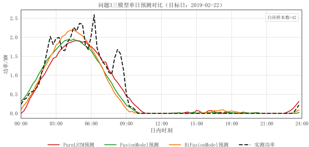
图 3: 气象预报融合链路预测曲线
