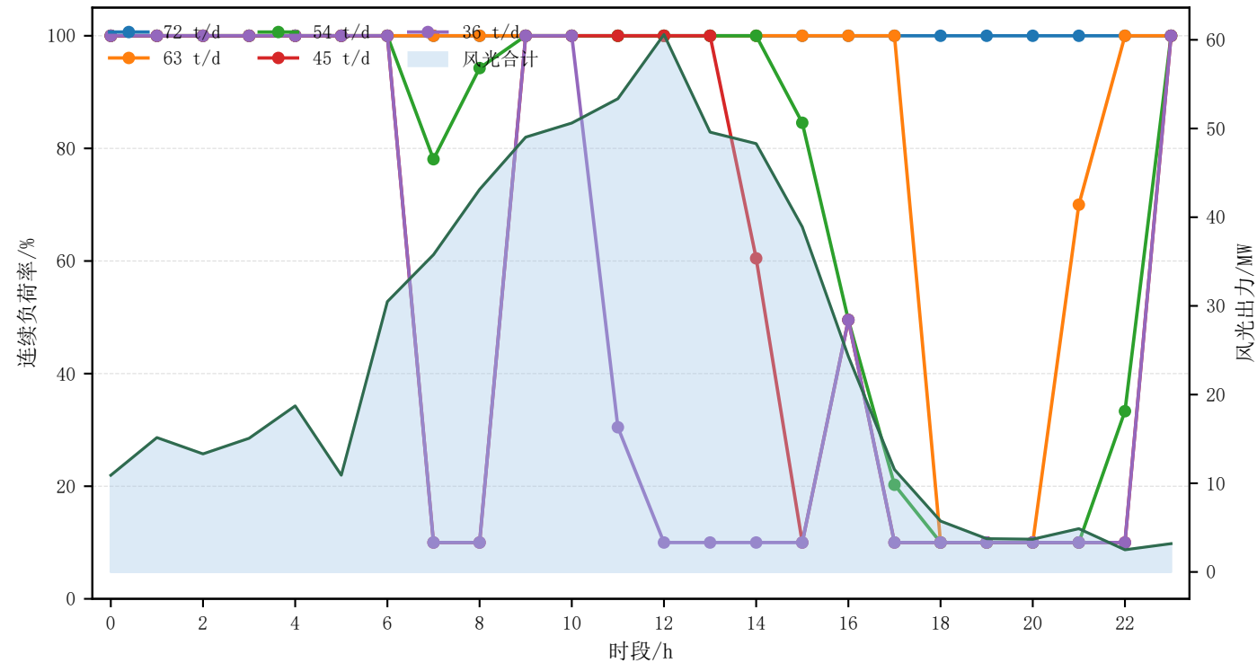
典型风光场景下连续制氨负荷率与风光出力
