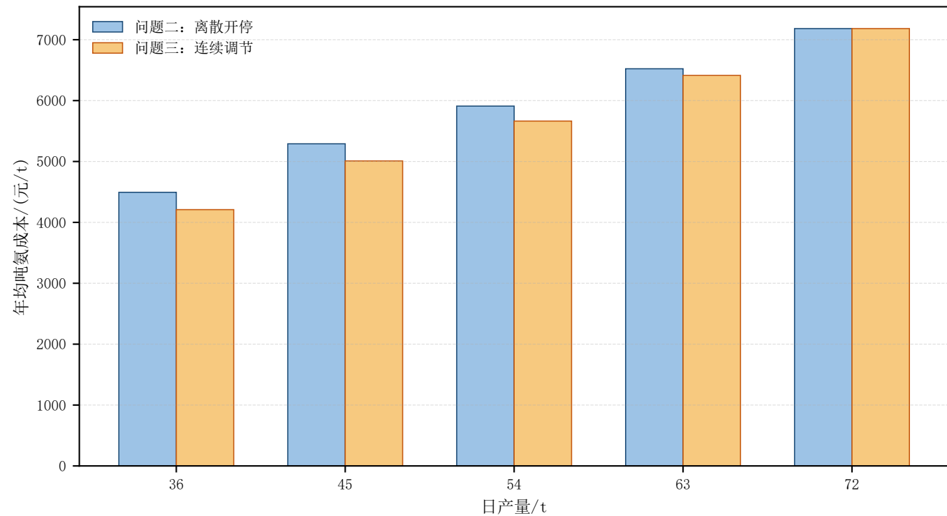
离散开停与连续调节的年均吨氨成本对比
