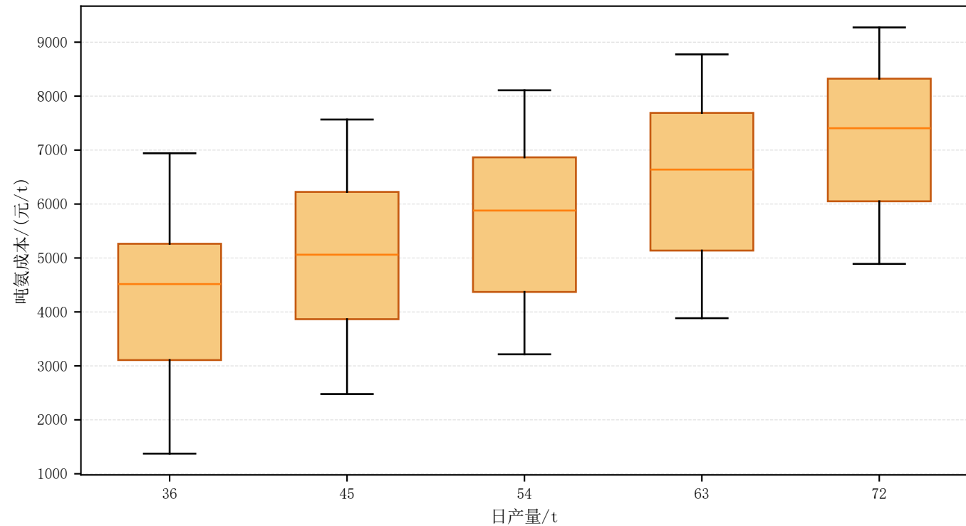
连续调节下24种风光场景吨氨成本分布
