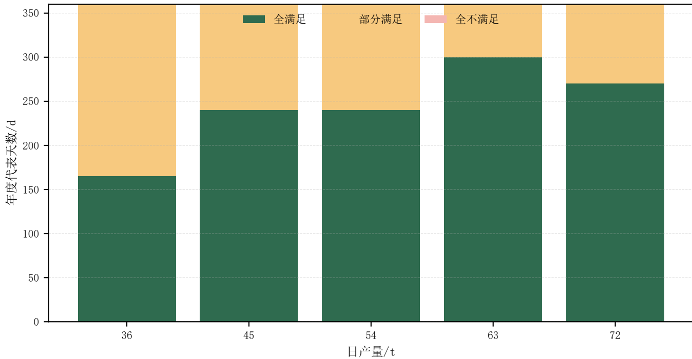
连续调节下年度绿电指标合格类型统计
