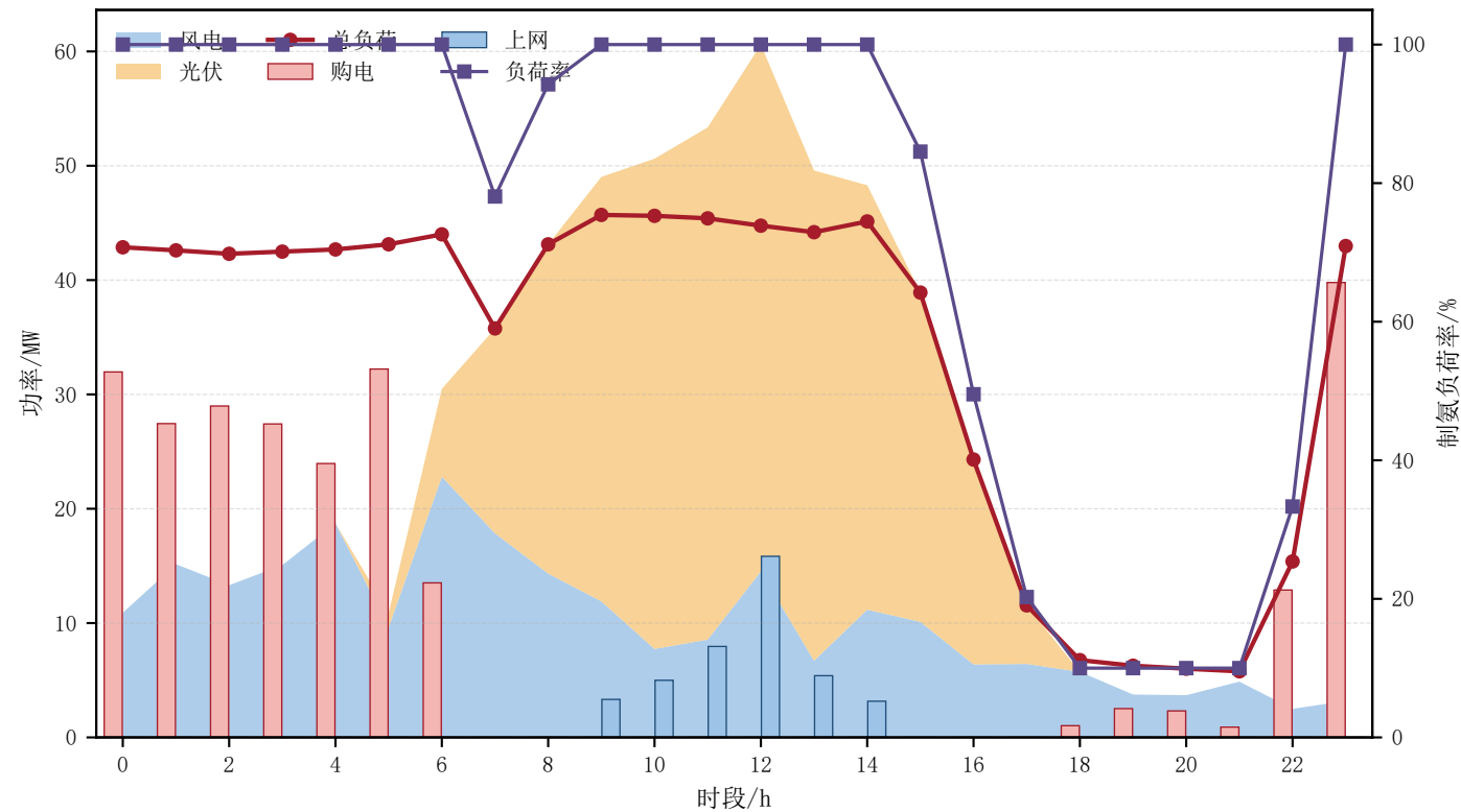
典型场景连续调节功率平衡 (54 t/d)
