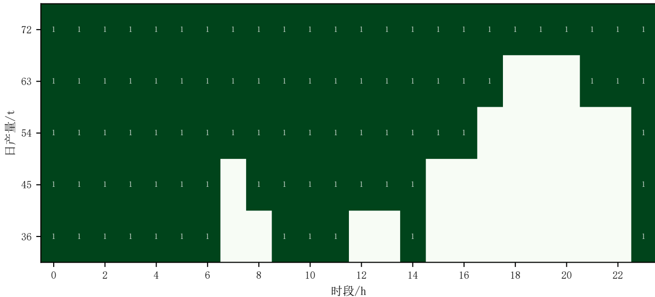
典型风光场景下不同日产量的最优开机时段
