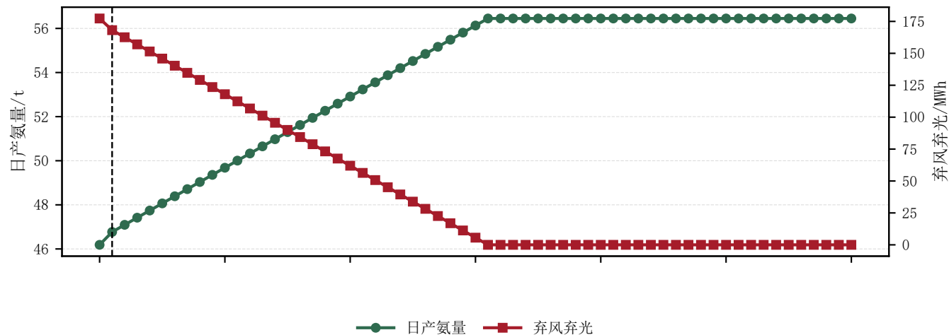
最大弃电场景下储能容量扫描结果
