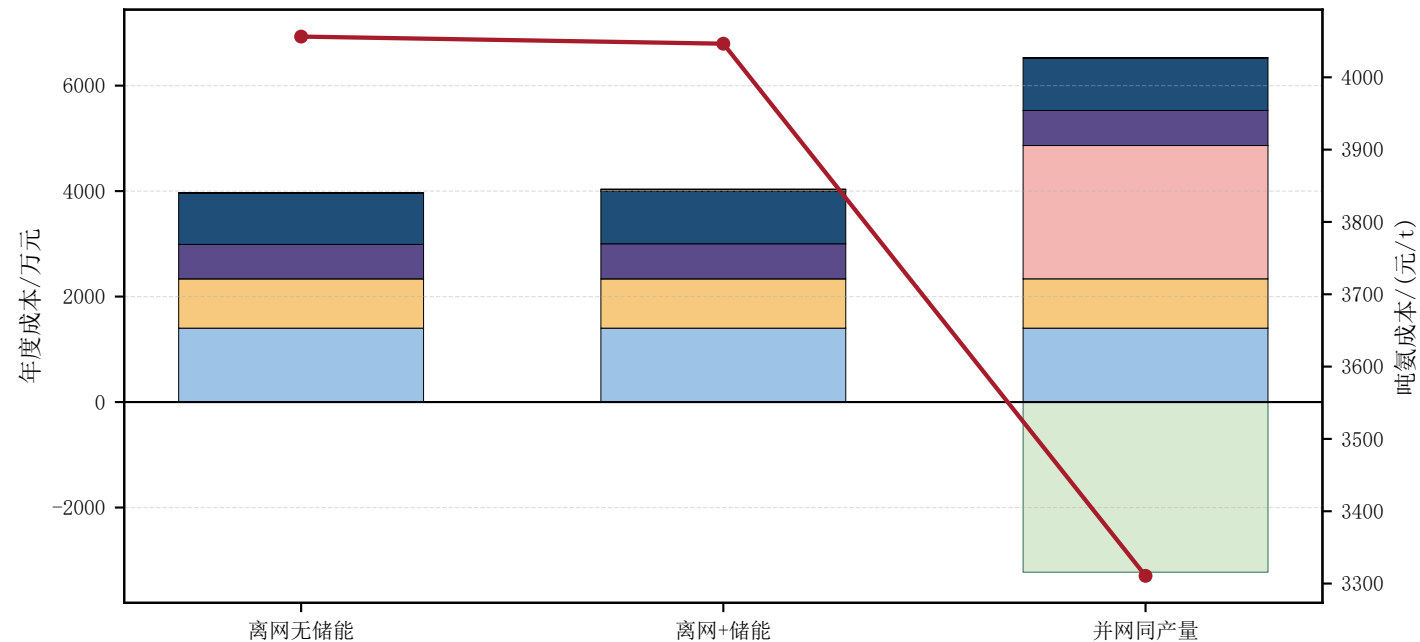
离网与并网同产量方案年度成本分项对比
