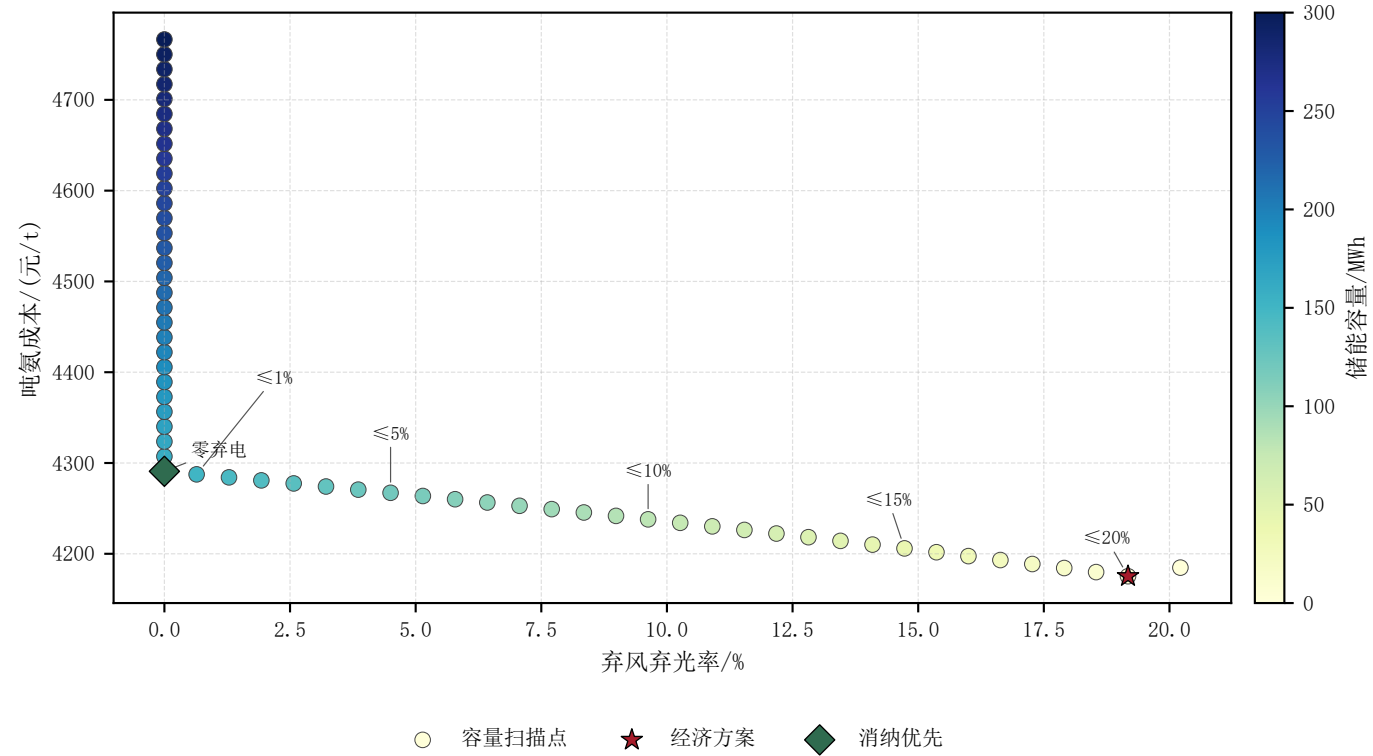
最大弃电场景储能容量的成本-消纳权衡
