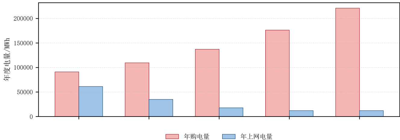
连续调节下日产量对电网交换和指标合格性的影响
