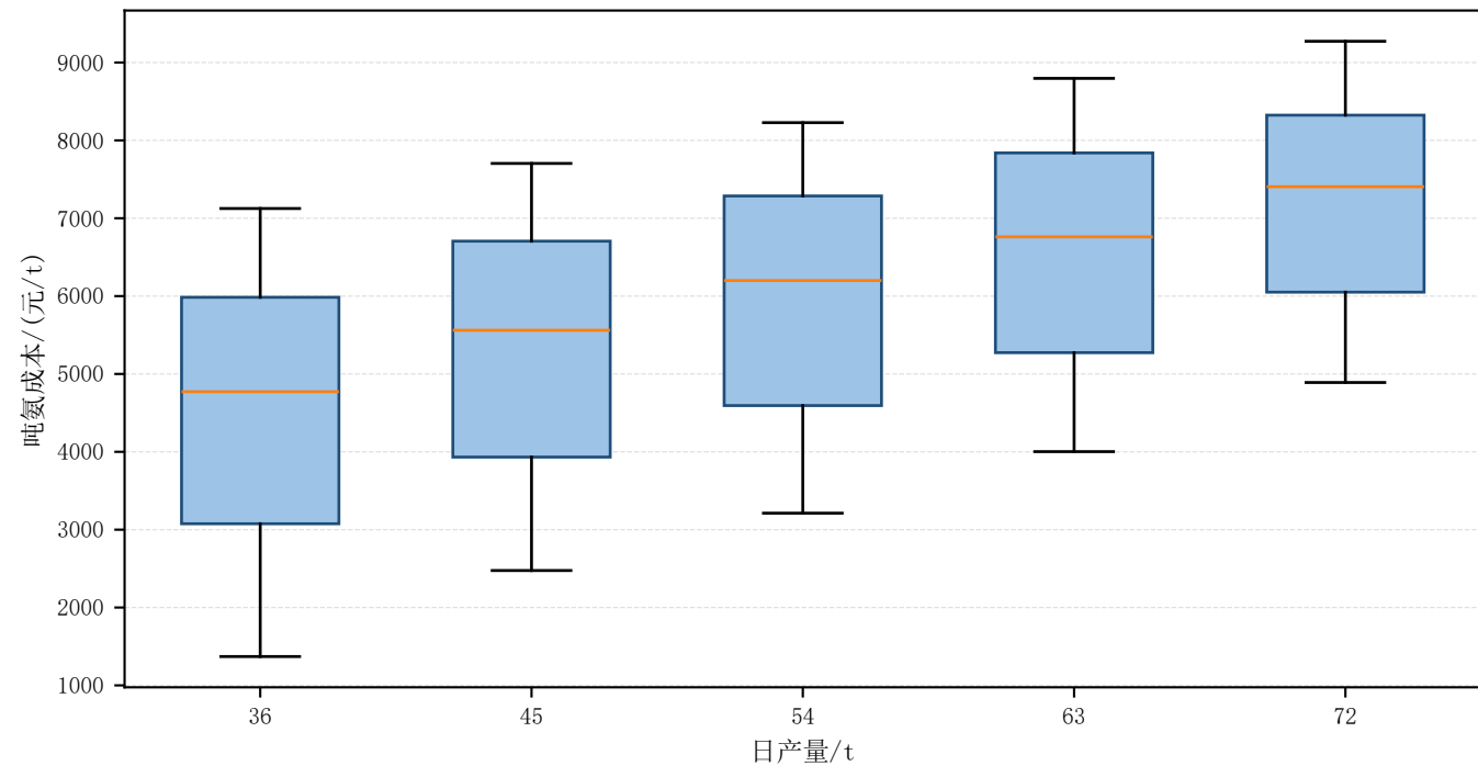
24种风光场景下吨氨成本分布
