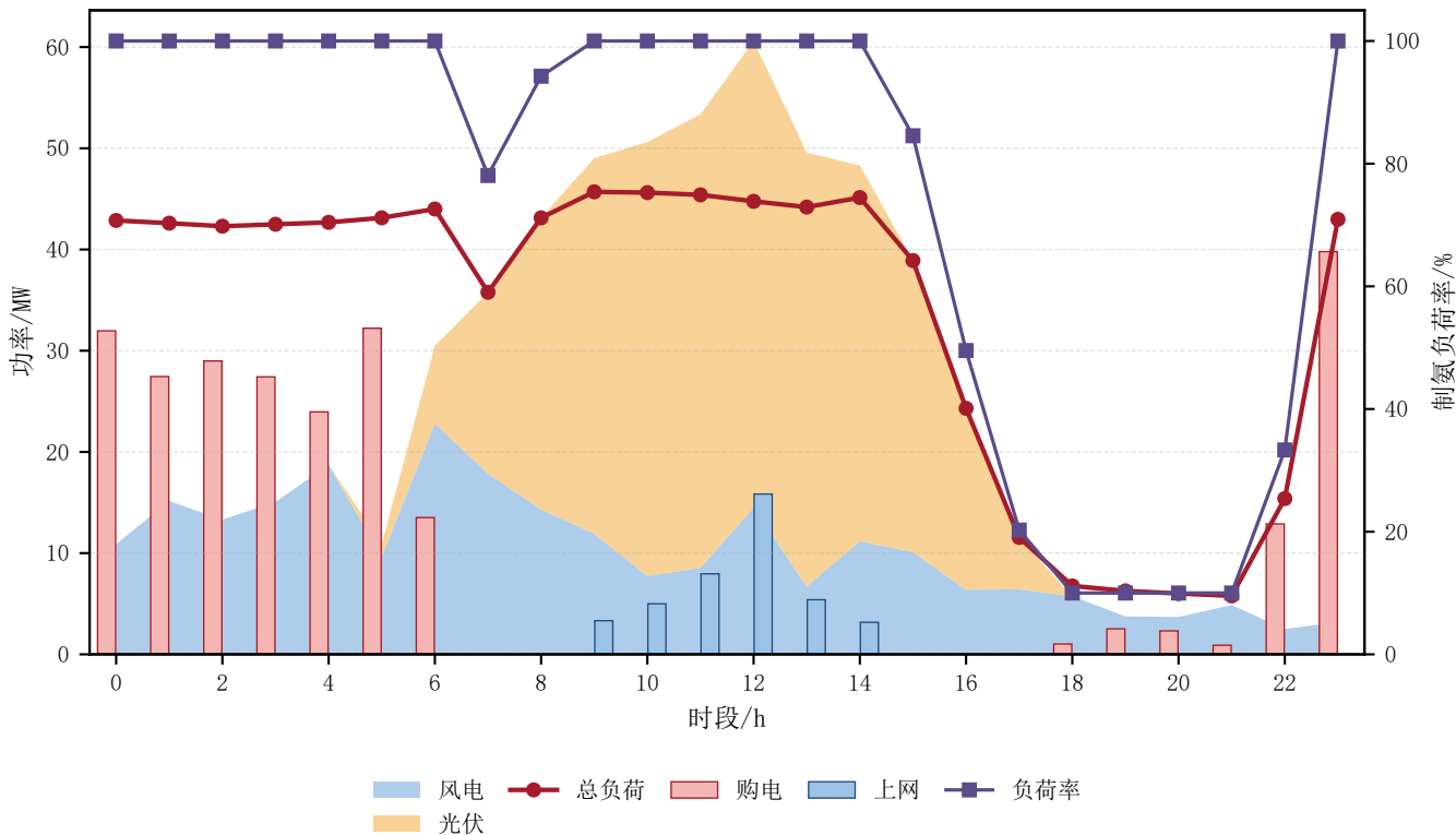
典型场景连续调节功率平衡 (54 t/d)
