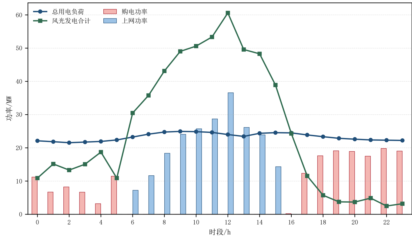
典型日功率平衡与购售电功率
