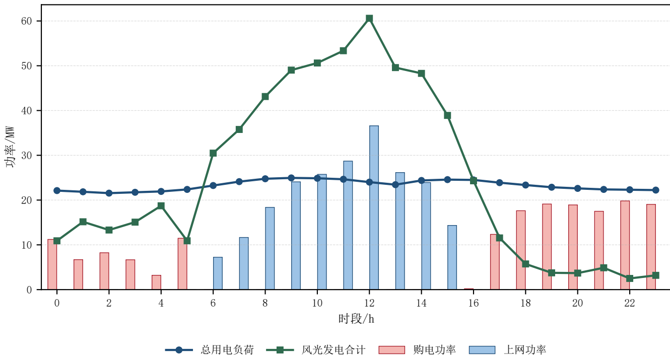
典型日功率平衡与购售电功率
