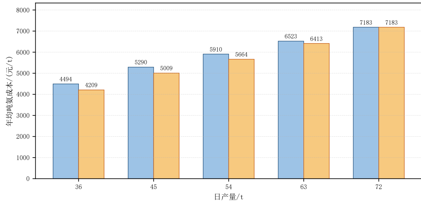
离散开停与连续调节的年均吨氨成本对比
