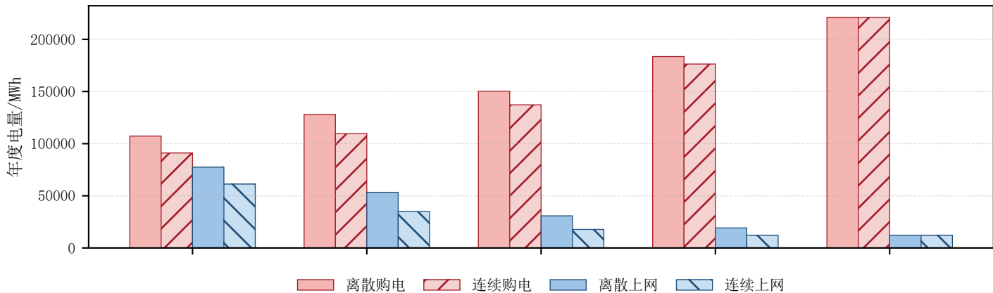
离散开停与连续调节的购售电和绿电指标对比
