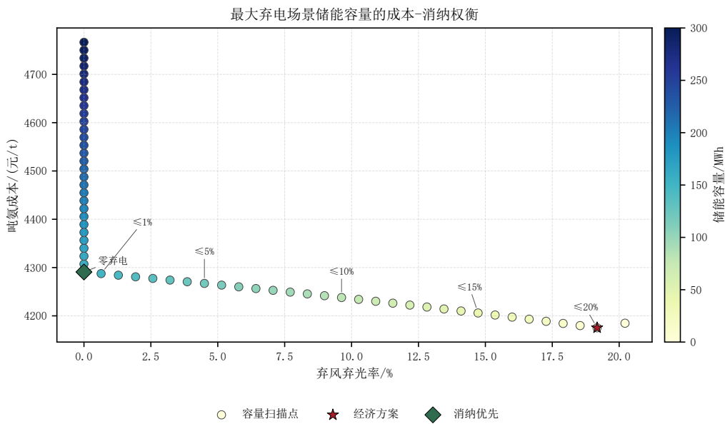
图 5：最大弃电场景储能容量的成本-消纳权衡
