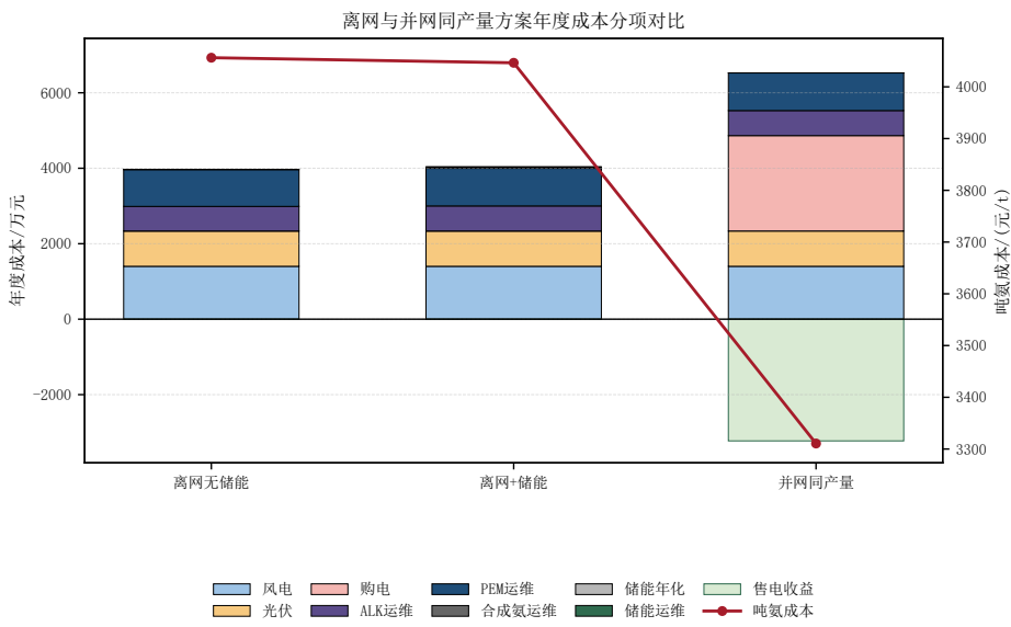
图 6：离网与并网同产量的成本分项对比
