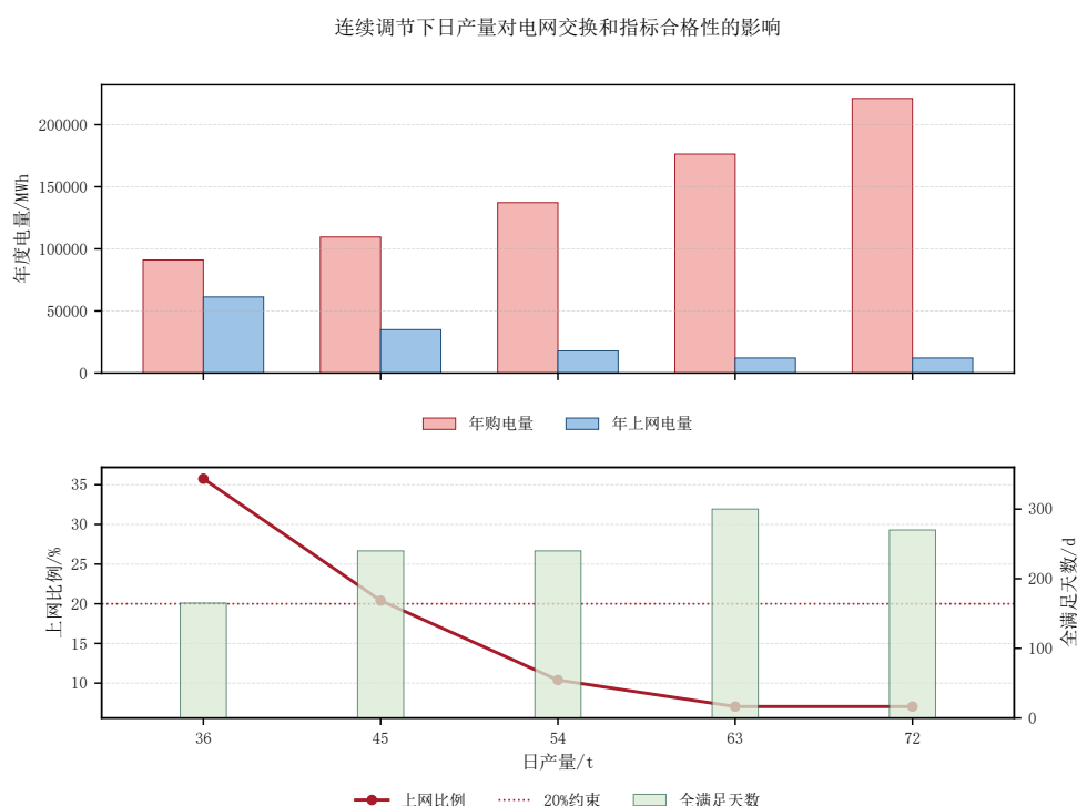
图 7：连续调节下日产量对电网交换和指标合格性的影响
