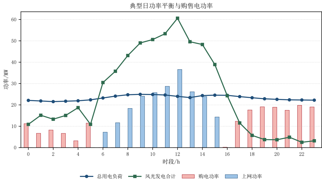
图 1: 典型日风光出力、园区负荷与电网交换功率
