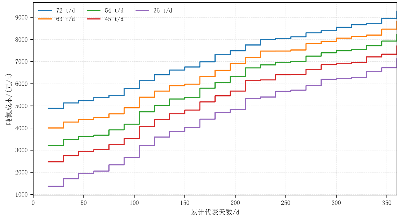
全年代表场景吨氨成本分布曲线
