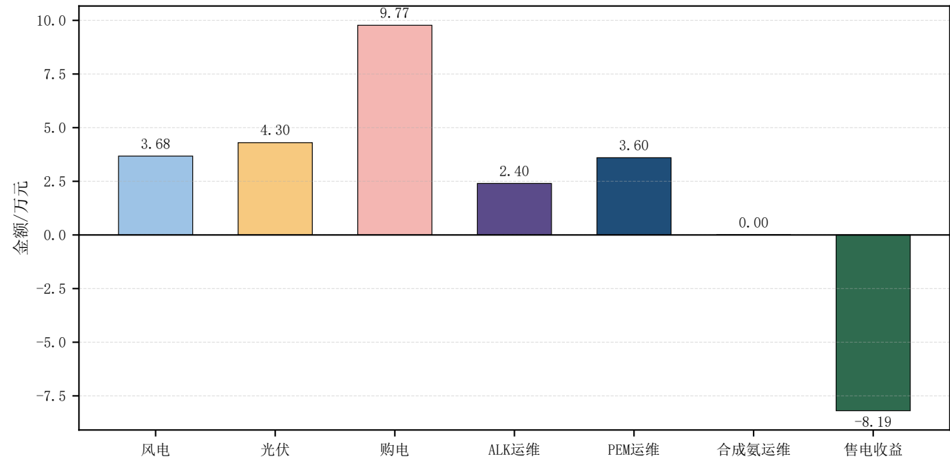
典型日成本与收益分项
