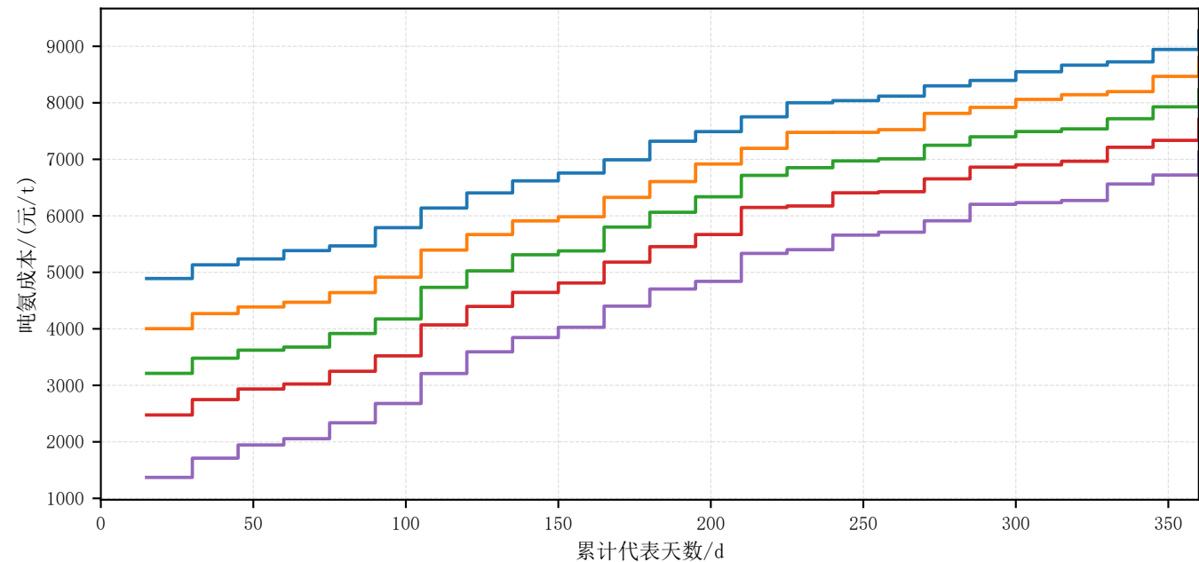
全年代表场景吨氨成本分布曲线
