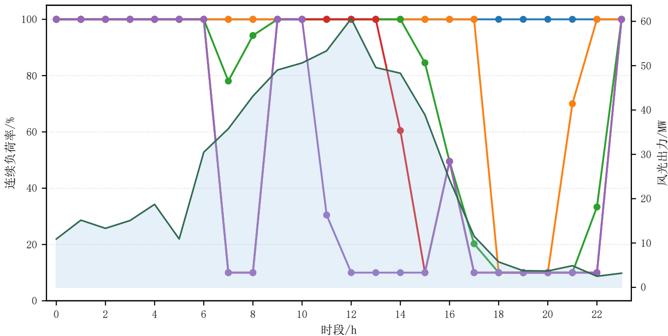
典型风光场景下连续制氨负荷率曲线
