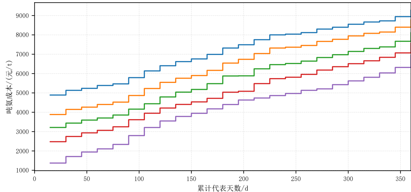
连续调节下全年代表场景吨氨成本分布曲线
