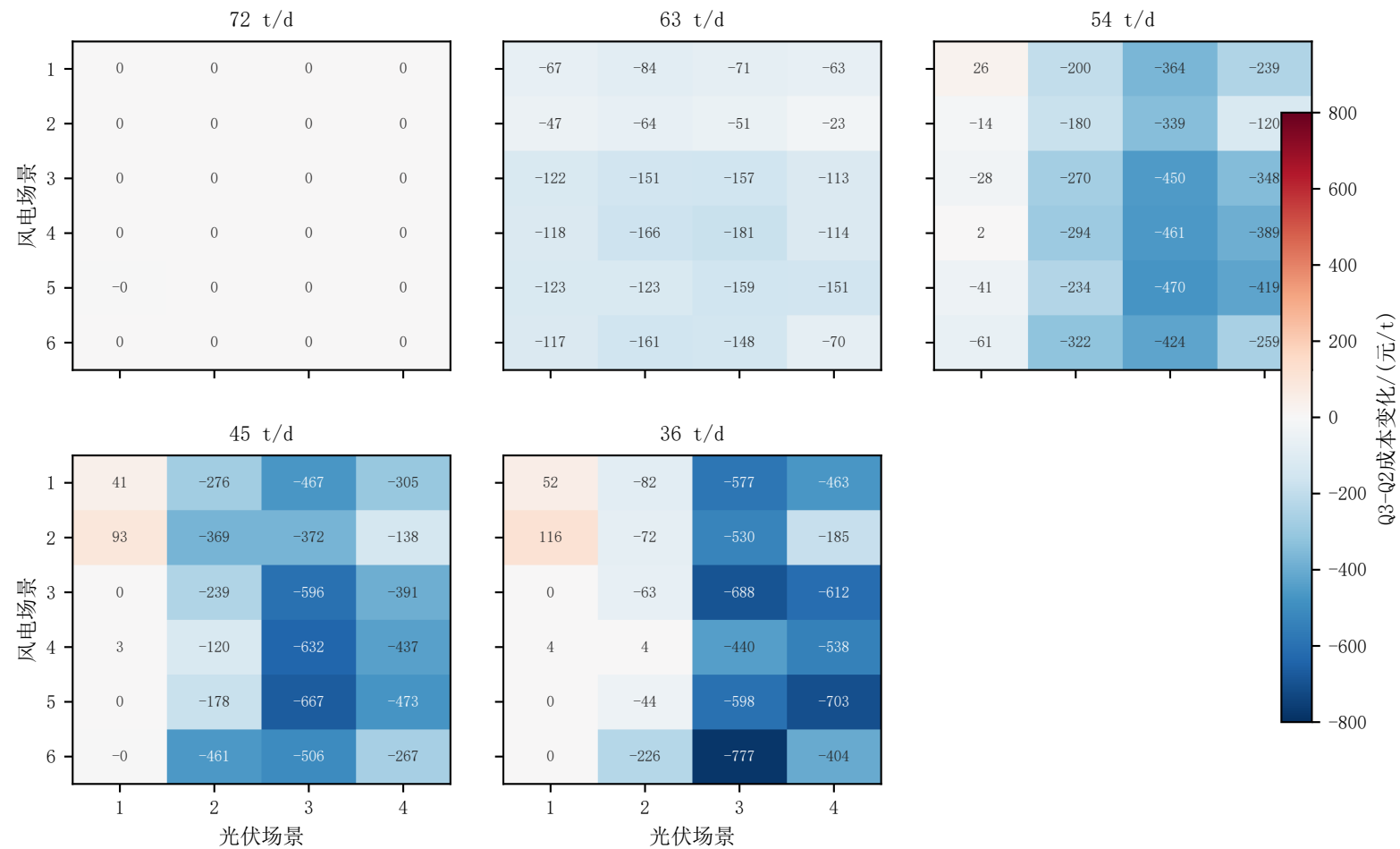
连续调节相对离散开停的场景吨氨成本变化
