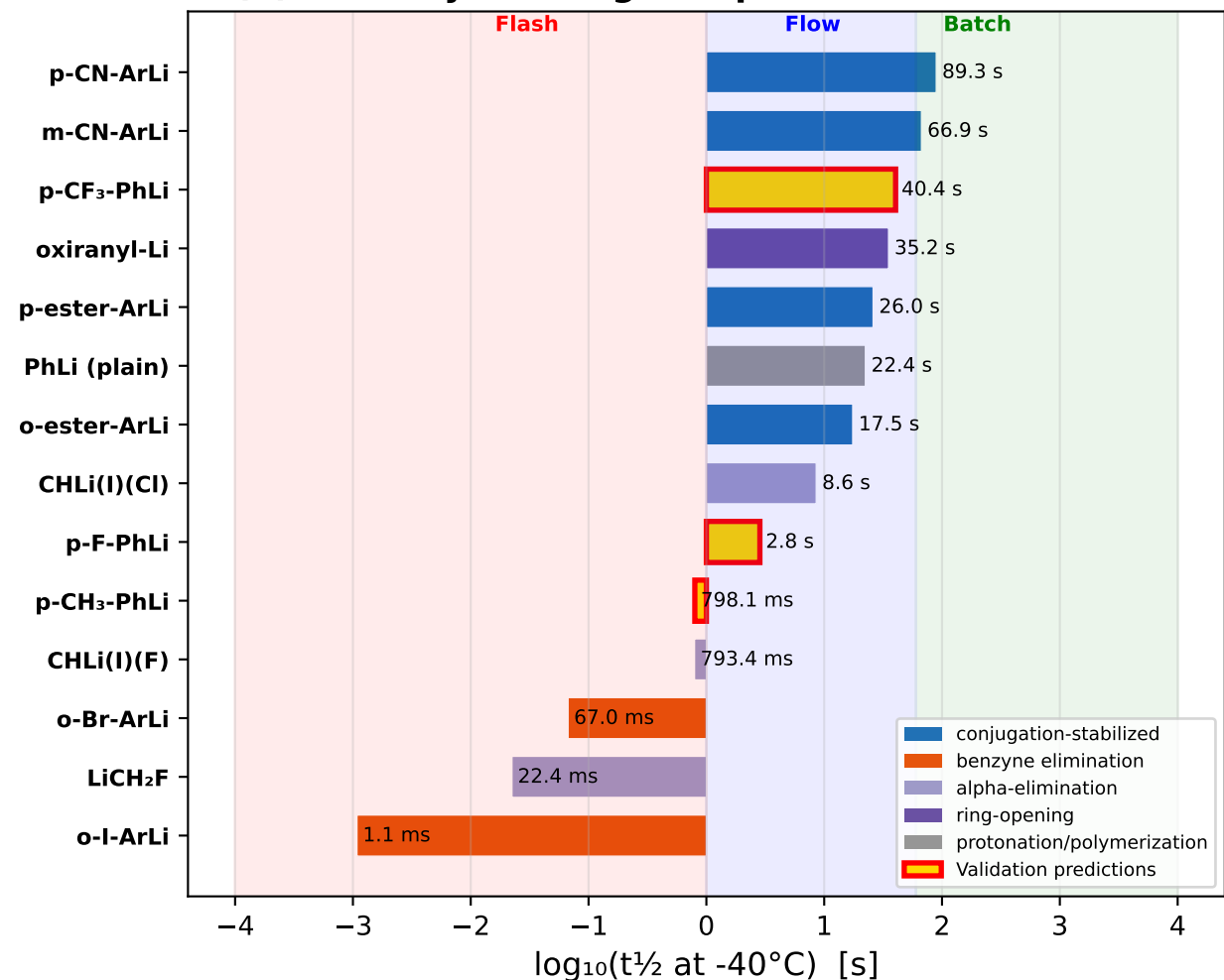
(d) Stability Ranking + Experimental Predictions
