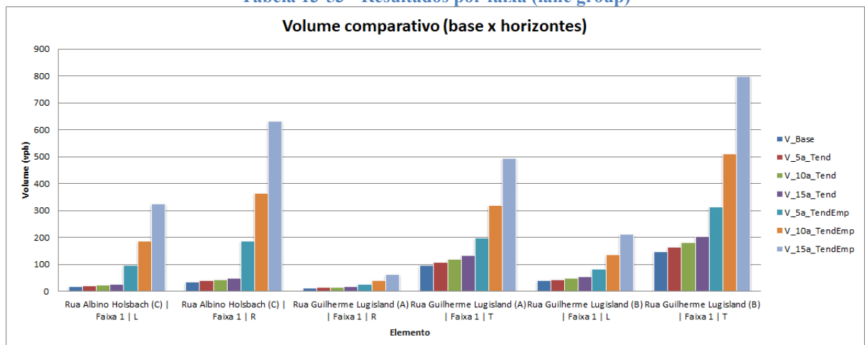
Gráfico 13-25 - Volume comparativo
