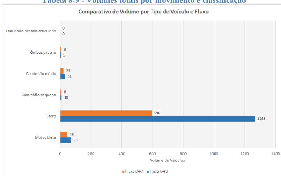
Gráfico 8-5 - Composição veicular
