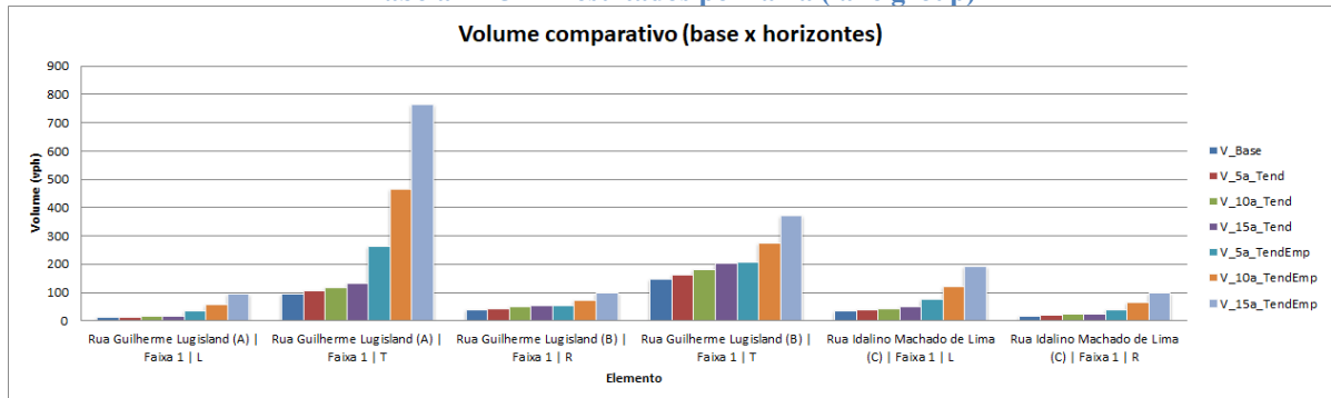
Gráfico 12-7 - Volume comparativo
