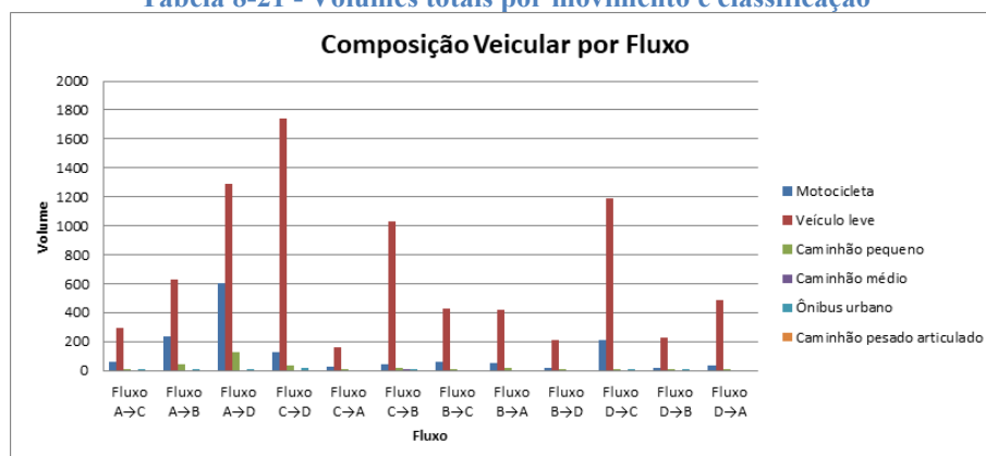
Gráfico 8-15 - Composição veicular
