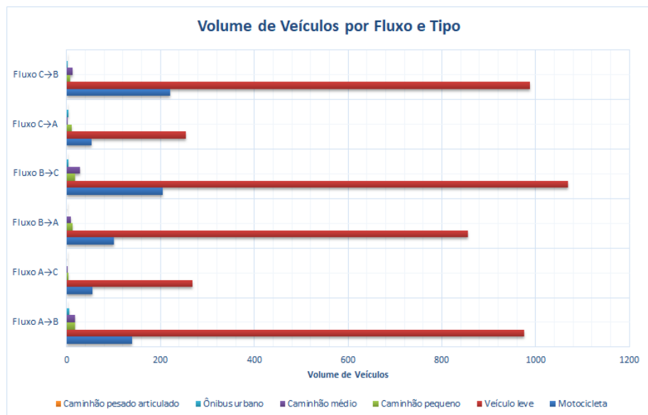
Gráfico 8-12 - Composição veicular
