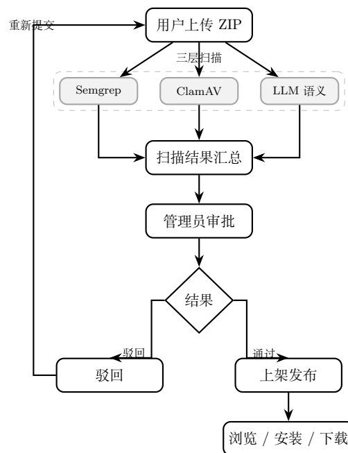
图 3: Skill 完整生命周期流程
