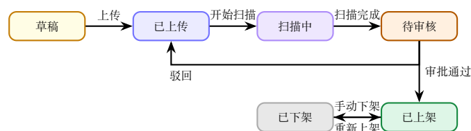
图 4：上架与下架状态机
