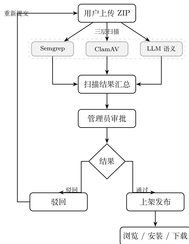
图 3: Skill 完整生命周期流程
