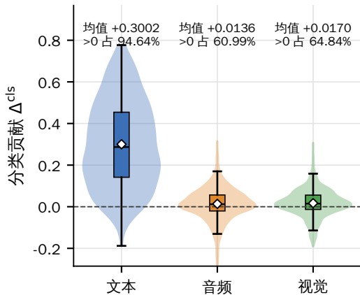
(a) 分类输出 (n=728, \diamond 为均值)
